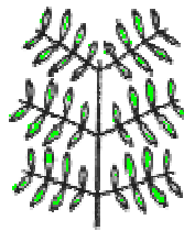
mehrfach gefiedert
