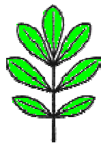
unpaarig gefiedert
