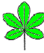
gefingert
