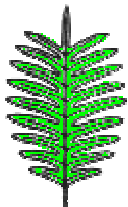
kammförmig
