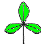
dreizählig
