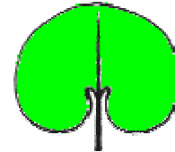
nierenförmig
