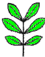
paarig gefiedert
