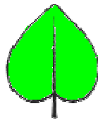
herzförmig
