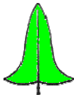
spießförmig
