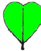
verkehrt herzförmig
